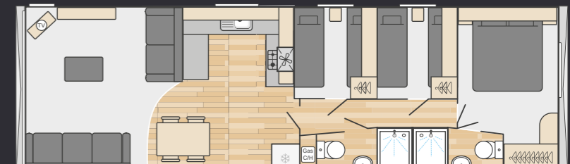
39' x 12' ES - 3 Bedroom
